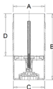
Oval Top Fill
